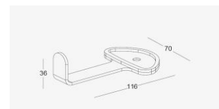
Wandabstandhalter
